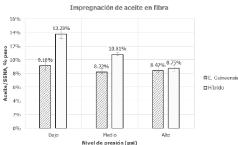
Figura 62. Impregnación de aceite en fibra a tres niveles de presión en prensas para material híbrido y guineensis .
