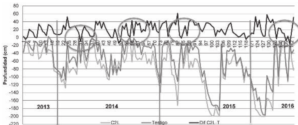
FIGURA 53. Fluctuación de niveles freáticos y épocas críticas por efecto de las mayores precipitaciones.
