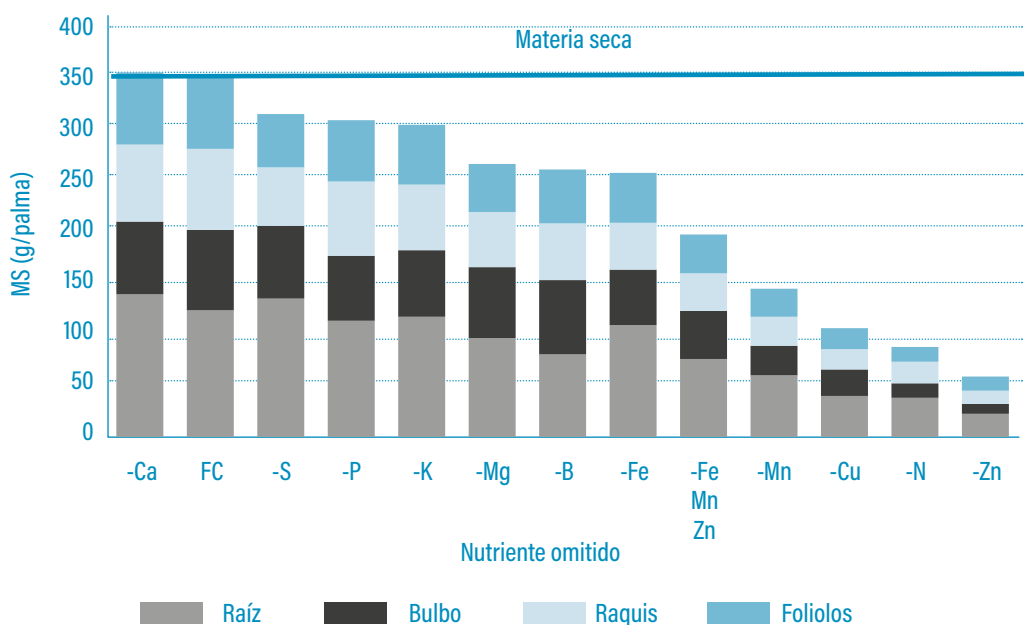
Figura 16. Acumulación de biomasa por componente de la planta, y en función de diferentes tratamientos de omisión de nutrientes
